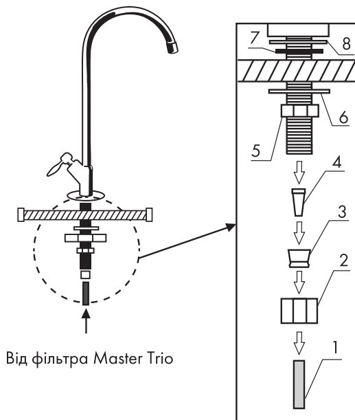
Рис. 1. Підключення проточного фільтра Organic Master Trio
