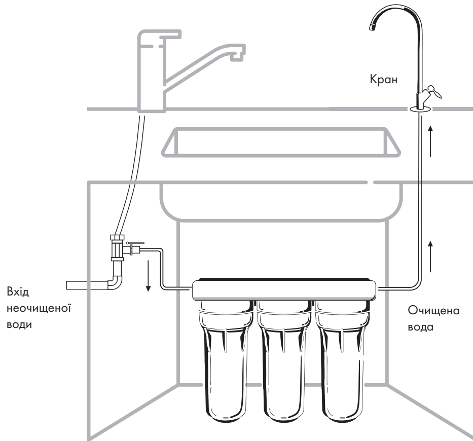
Рис. 2. Загальний вигляд підключеного фільтра Organic Master Trio
